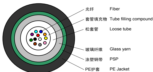
光缆结构图 Cable Structure
